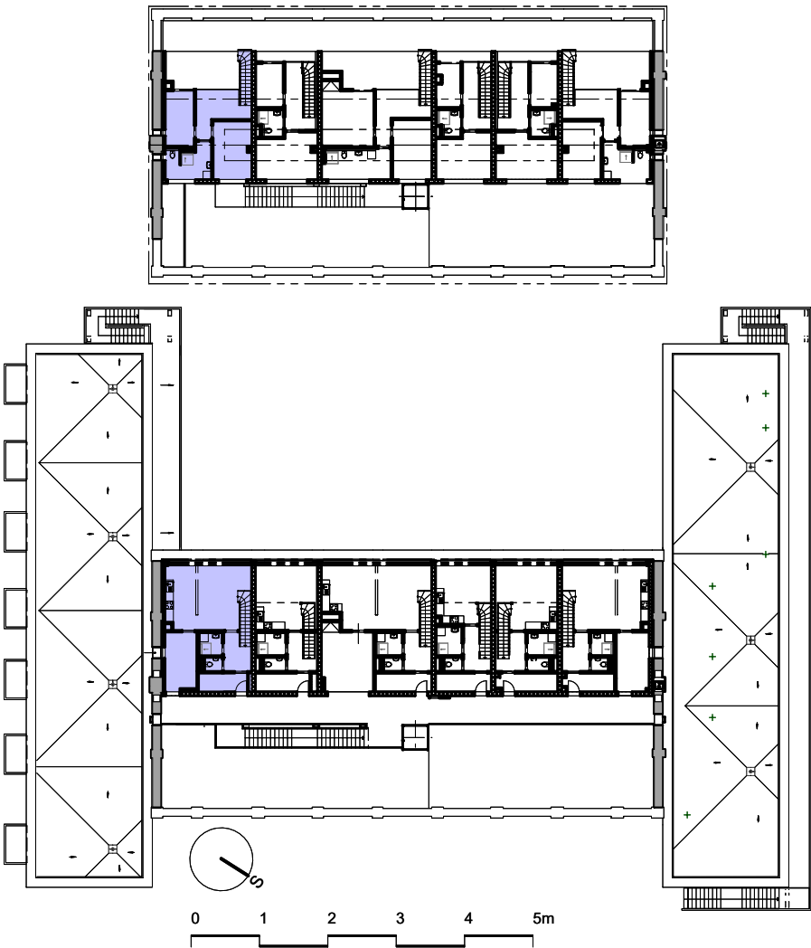
Schéma půdorys
